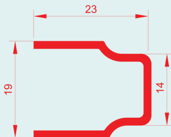
REFUERZO 501 R501
